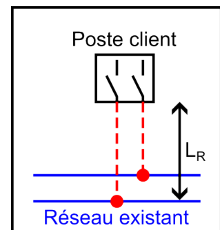
Raccordement en double dérivation
