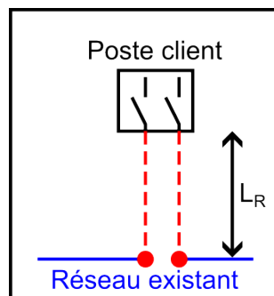
Raccordement en coupure d'artère
